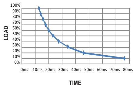
DDR-120D-12
